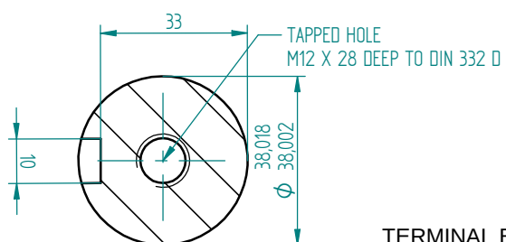
Przekrój A-A 1:1
